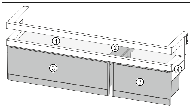
Fig. 76 Primjer izgleda police u vratima s kutijama VarioBox (1) Polica (2) Pridržni dio za VarioBoxove (3) VarioBoxovi (4) Bočni dio
